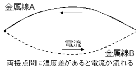
図4 熱電対の計測原理
