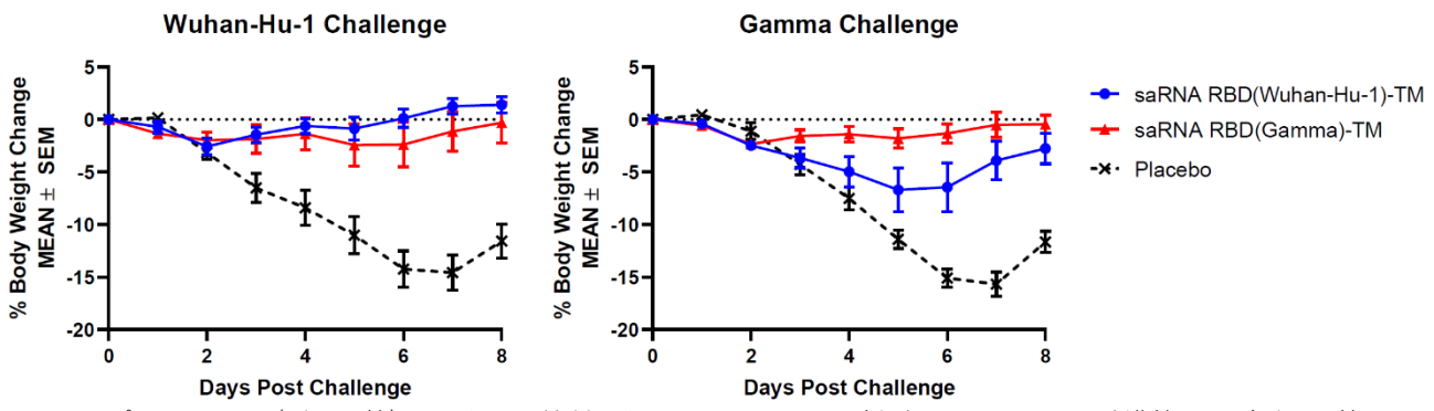
図 3. レプリコン RBD(ガンマ株)-TM を 2 回接種したハムスターでは、新型コロナウイルス武漢株およびガンマ株での攻撃接種後に大きな体重変化は確認されなかった
