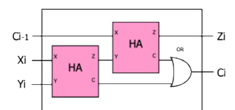
図C なぜこれが足し算器?
