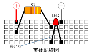
実体配線図
