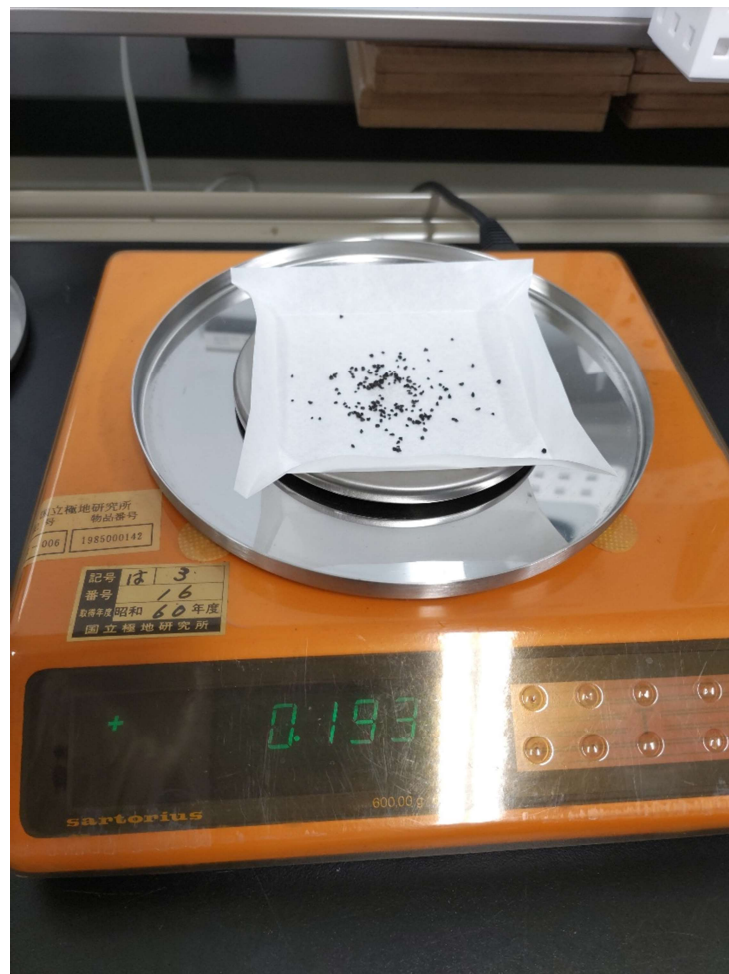
図1：衝撃実験に用いたオルゲイユ隕石の試料
