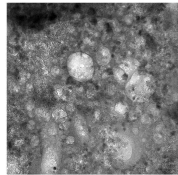
図 4：リュウグウ粒子と衝撃実験後の隕石試料に見られる衝突の痕跡（電子顕微鏡写真）
