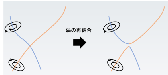
図 2 量子渦の再結合の模式図。接触した 2 本の量子渦が互いに繋ぎ変えた後に、急速に離れていく。
