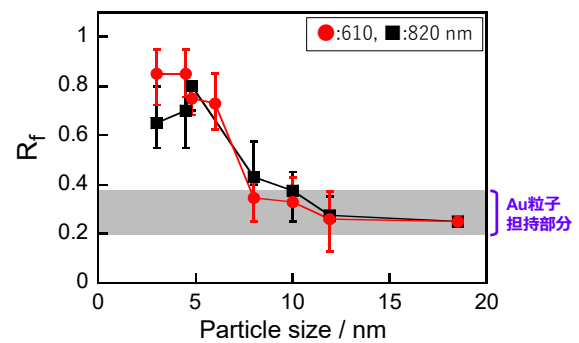
図 4 プラズモン TLC を用いたサイズの異なる ZAIS 量子ドットの光捕捉。照射単色光波長: 610 nm および 820 nm。縦軸は、 R_f 値を示す【注 4) 参照】。
