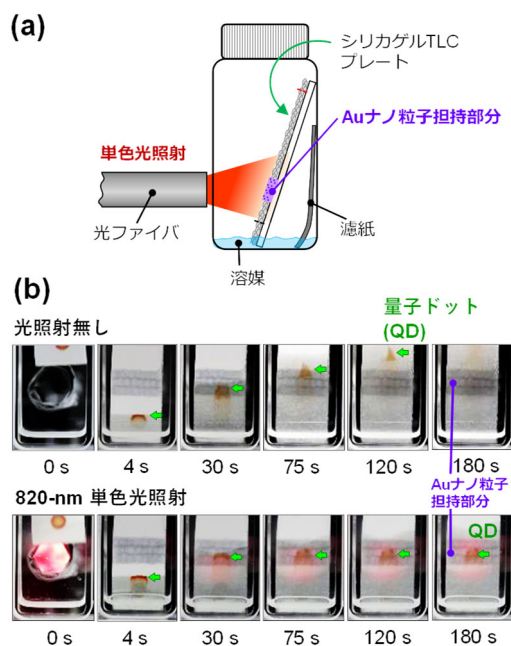
図2 (a) プラズモン TLC の実験装置の模式図。(b) プラズモン TLC プレート上を移動する ZAIS 量子ドット(サイズ: 19 nm)の時間変化。写真の下の数字は、溶媒が TLC プレートを上昇している時間(秒)。光照射無しで量子ドットを移動させても、Au ナノ粒子保持部分に捕捉されないが、820nm 単色光を照射しながら移動させると、Au 保持部分に選択的に光捕捉された。
