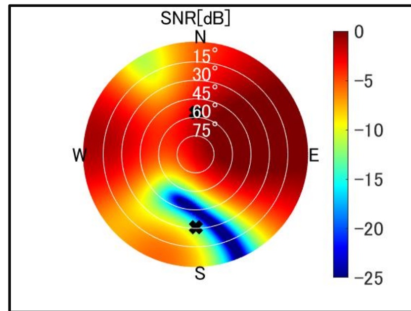
図2 アレーアンテナによる指向性制御の例
