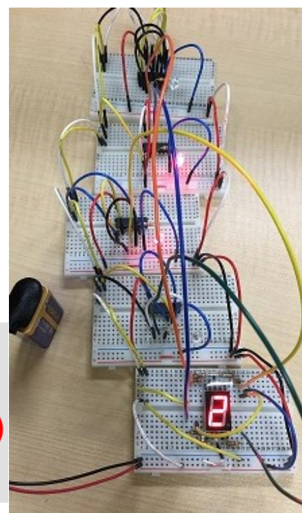
NANDを組合わせて2進数を10進数に! (論理回路実験講座)
