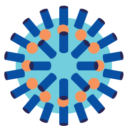
全粒子
