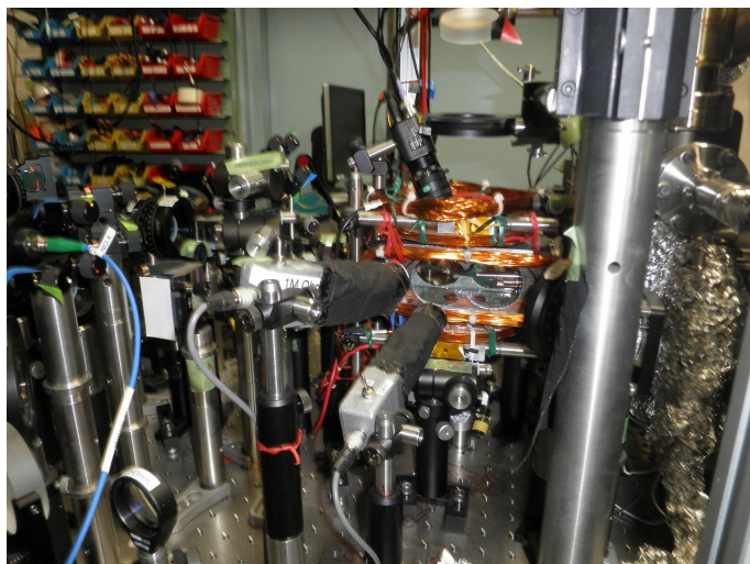
図 4.15: 1st MOT の光学系の外観:
