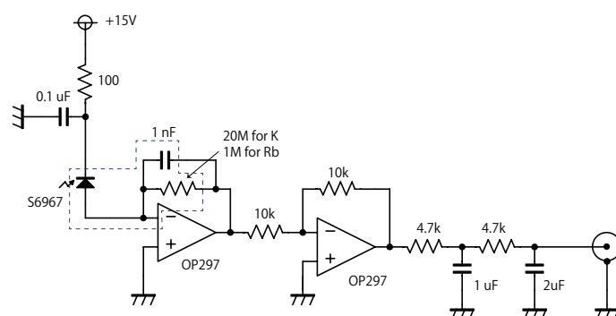
図 4.16: 蛍光観測の為の PD の回路図
