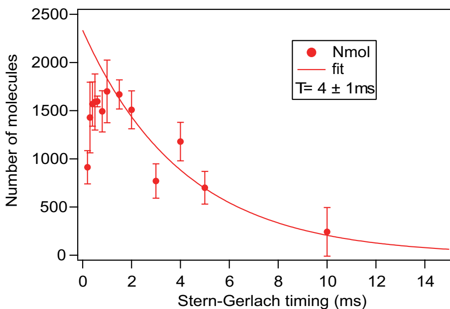
図 6.11: Stern-Gerlach のタイミングに対する生成分子数の変化
