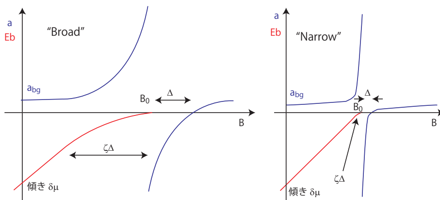
図 2.4: フェッシュバッハ共鳴近傍での散乱長と束縛エネルギー:
