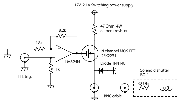
図 4.7: シャッタードライバー回路図
