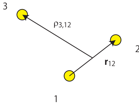
図 2.6: ヤコビ座標の例
