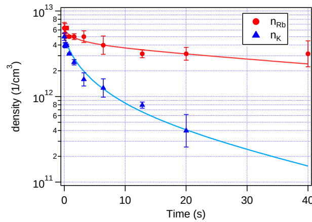
図 5.1: 三体ロス係数の測定 (吸収イメージング、 a = 250\text{ }a_0 ) : 青三角が K の密度、赤丸が Rb の密度を示す。青、赤の実線は \tau_\text{K} = 24\text{ s} 、 \tau_\text{Rb} = 130\text{ s} 、 L_\text{KKRb} = 7 \times 10^{-27}\text{ cm}^6/\text{s} 、 L_\text{KRbRb} = 0\text{ cm}^6/\text{s} での K、Rb 原子の密度の時間発展をシミュレーションしたものである。
