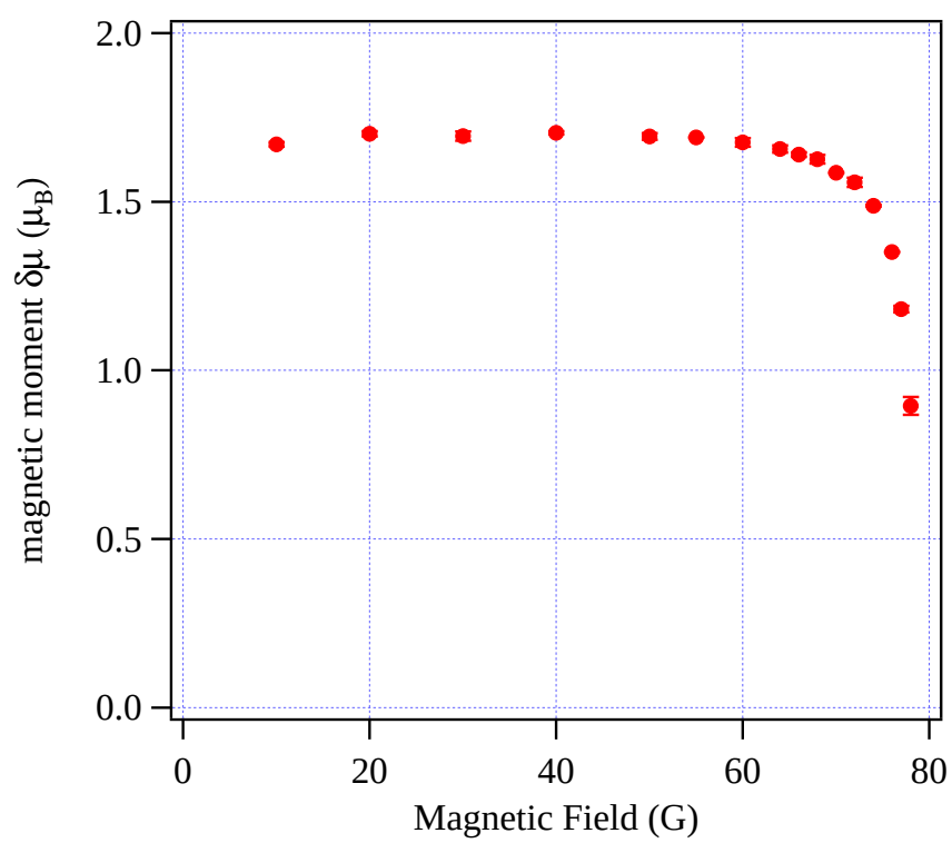
図 6.21: 分子の磁気モーメント \delta\mu の磁場依存性
