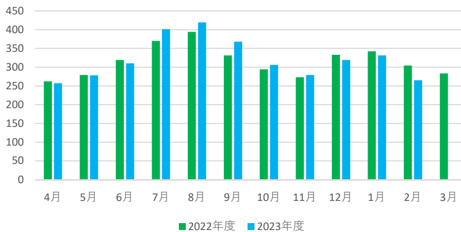
理学部A～D棟 電気使用量(MWh/月)
